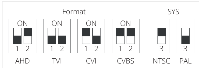
DIP-Schalter zur Wahl des Video-Ausgangs
